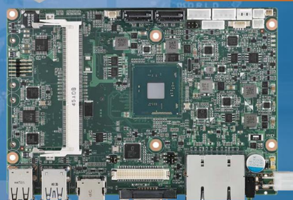
PCM-9310主板
