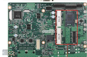
1个Mini PCIe支持SIM 1个mini PCIe支持MSATA
